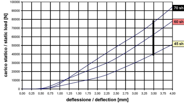
dimensioni 450 x 450 x 10,6 STRIPES PAD GG4545
