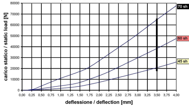
dimensioni 225 x 225 x 10,6 STRIPES PAD GG2222
