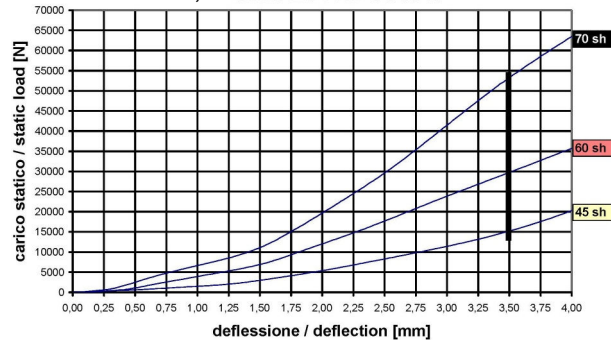
dimensioni 90 x 450 x 10,6 STRIPES PAD GG0945
